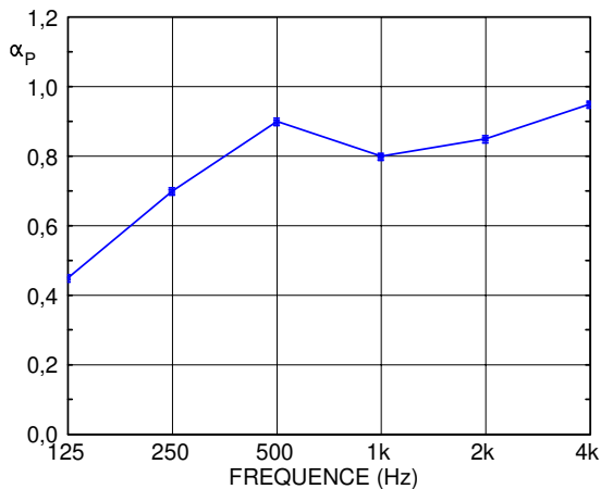
COEFFICIENT D'ABSORPTION ACOUSTIQUE linea 2.9.13 - MOYENNE DE 16 MESURES
