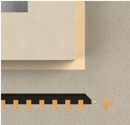
Etape 3 : Percer et coller le profil d'angle sur les contre-lattes
