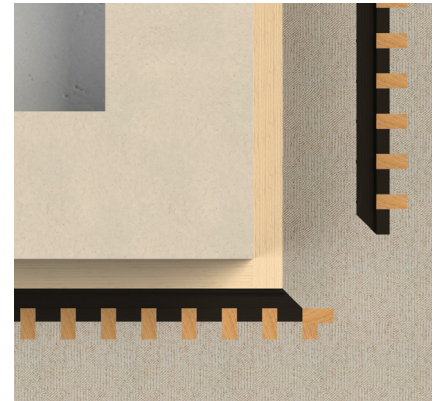
Etape 5 : Découper le panneau adjacent (idem étape 1)
