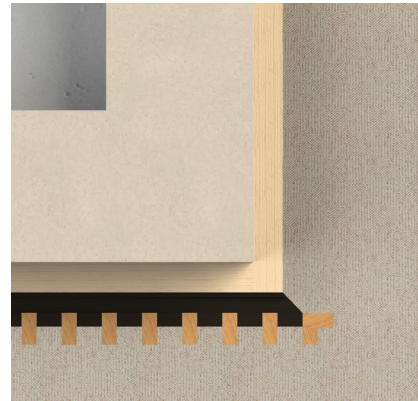
Etape 4 : Installer le panneau
